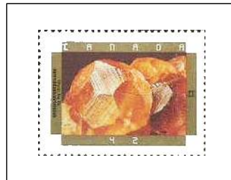
Grossulaire
