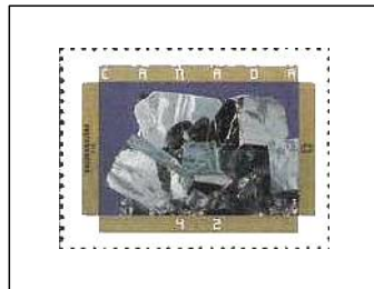
Galène
